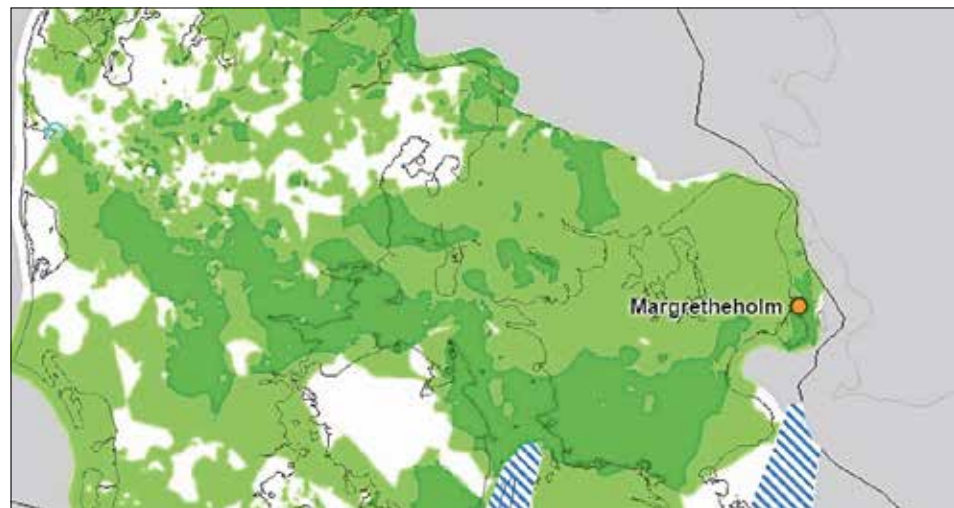
Kortet her viser de områder i Danmark, hvor der er potentiale for geotermiske anlæg. De hvide felter - eksempelvis store dele af Fyn - er uden mulighed for geotermi, men hele Nordsjælland ligger i lysegrøn, hvilket betyder, at der er et reservoir i undergrunden. Mørkegrøn er to eller flere reservoirer.
