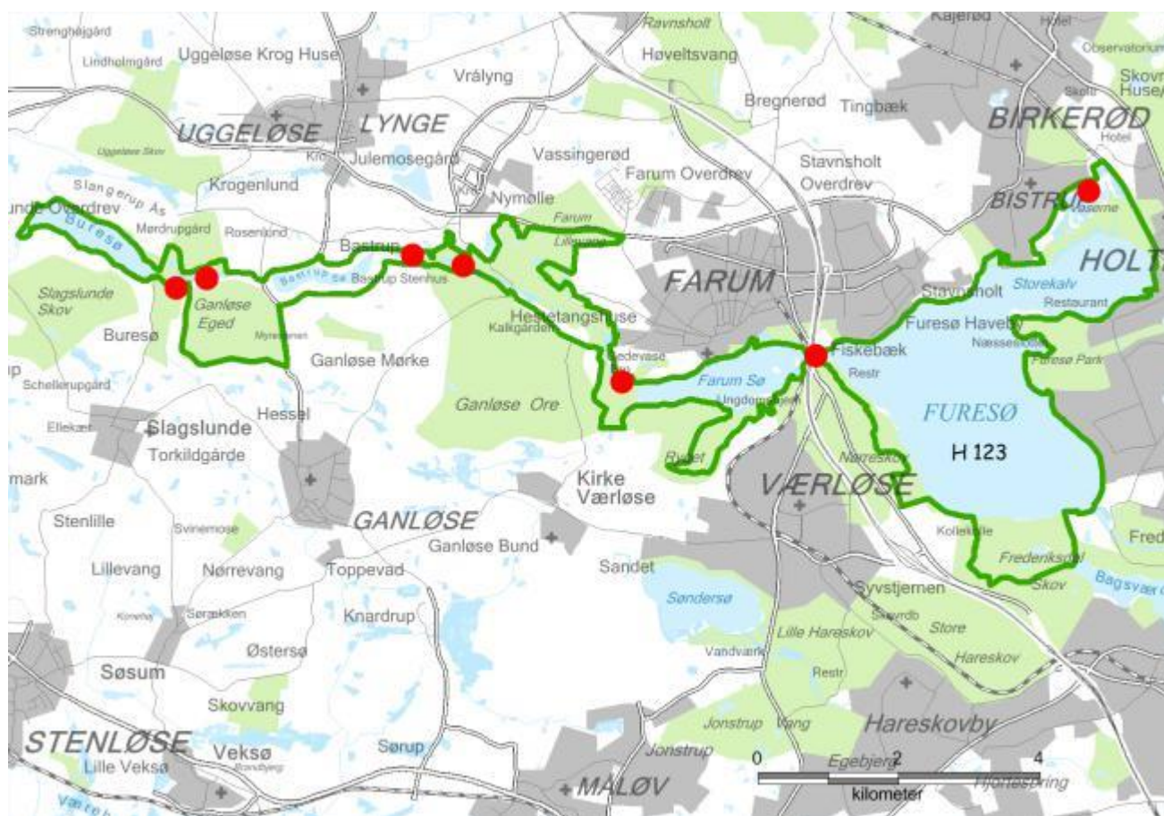
Overvåget forekomst af sumpvindelsnegl
