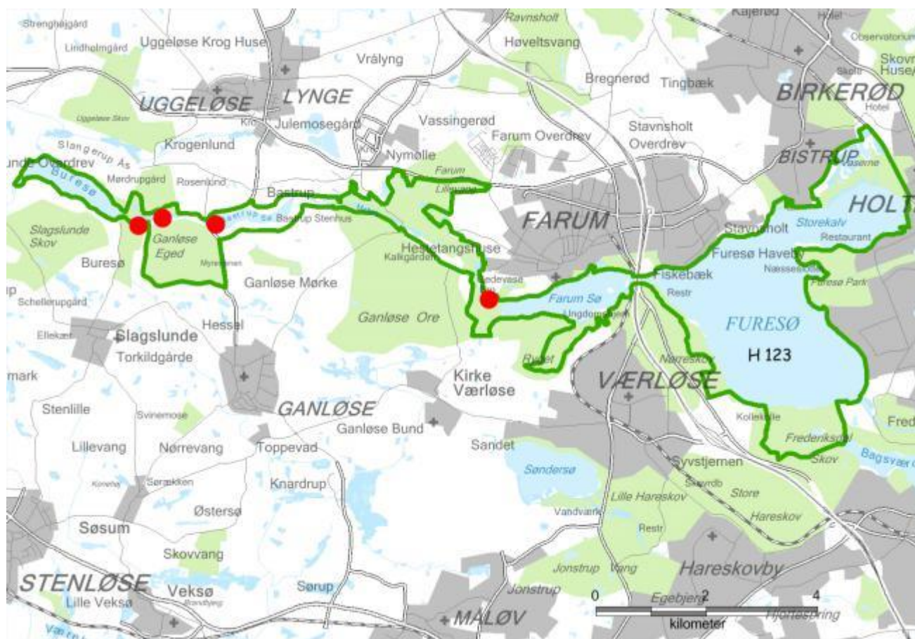
Overvåget forekomst af skæv vindelsnegl.
