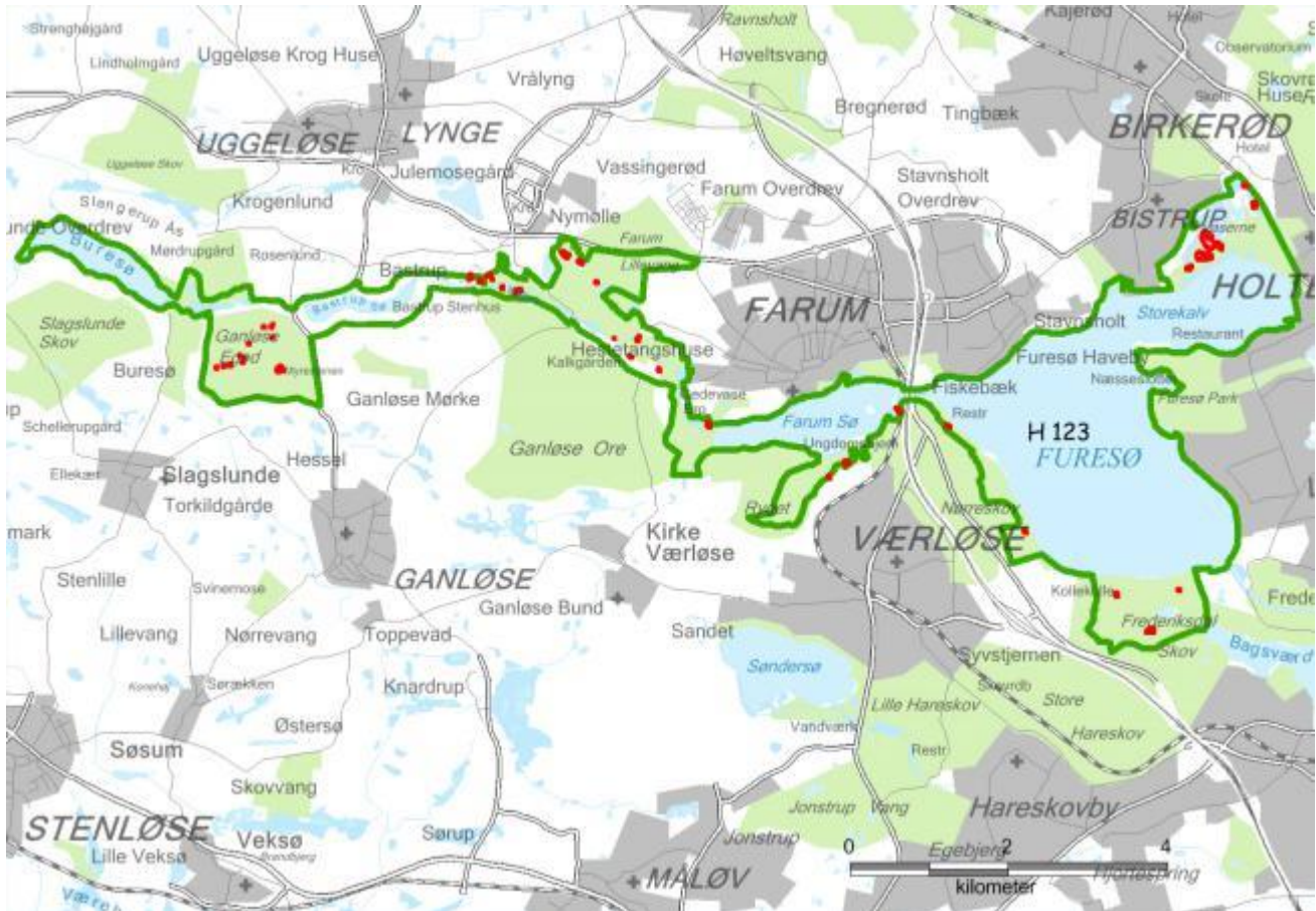
Kortlagte levesteder for stor vandsalamander
