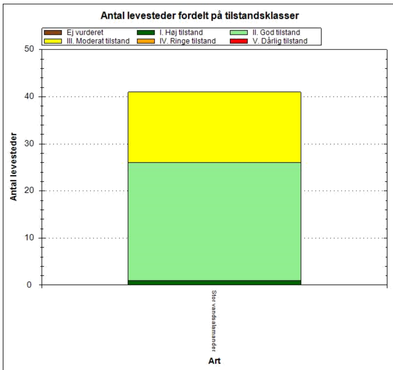
Tilstandsvurdering af områdets kortlagte levesteder.
