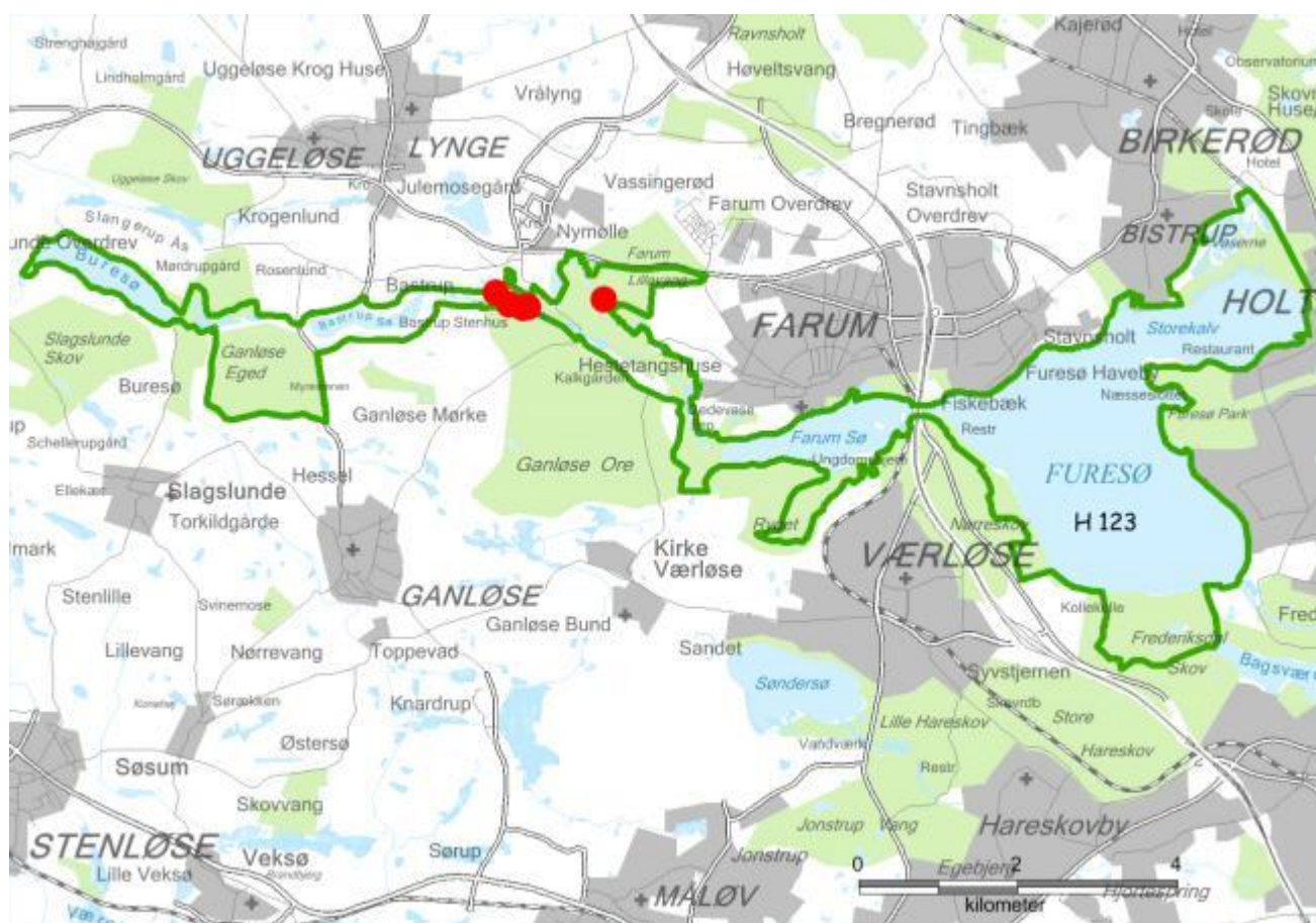
Overvåget forekomst af stor vandsalamander.
