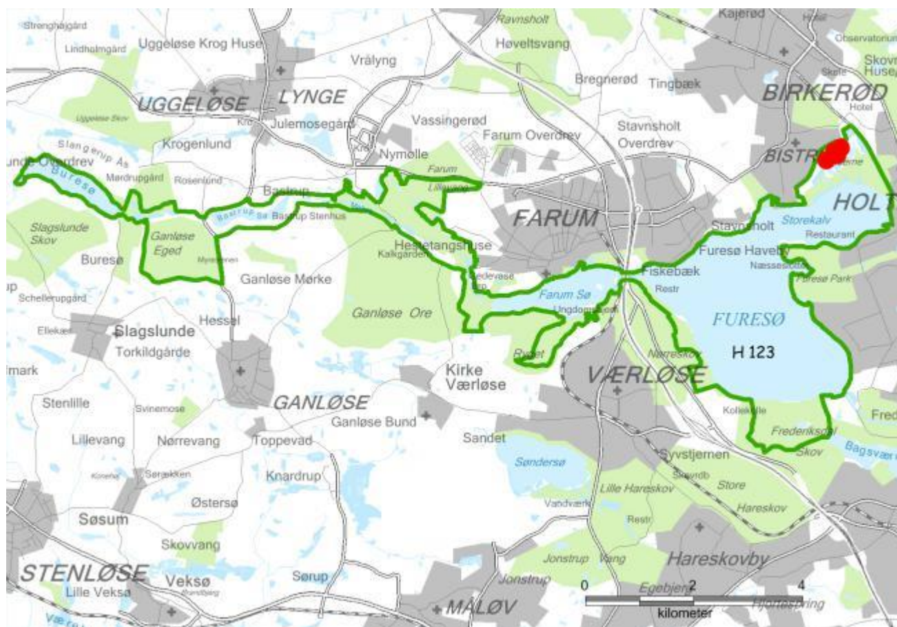
Overvåget forekomst af stor kær-guldsmed.
