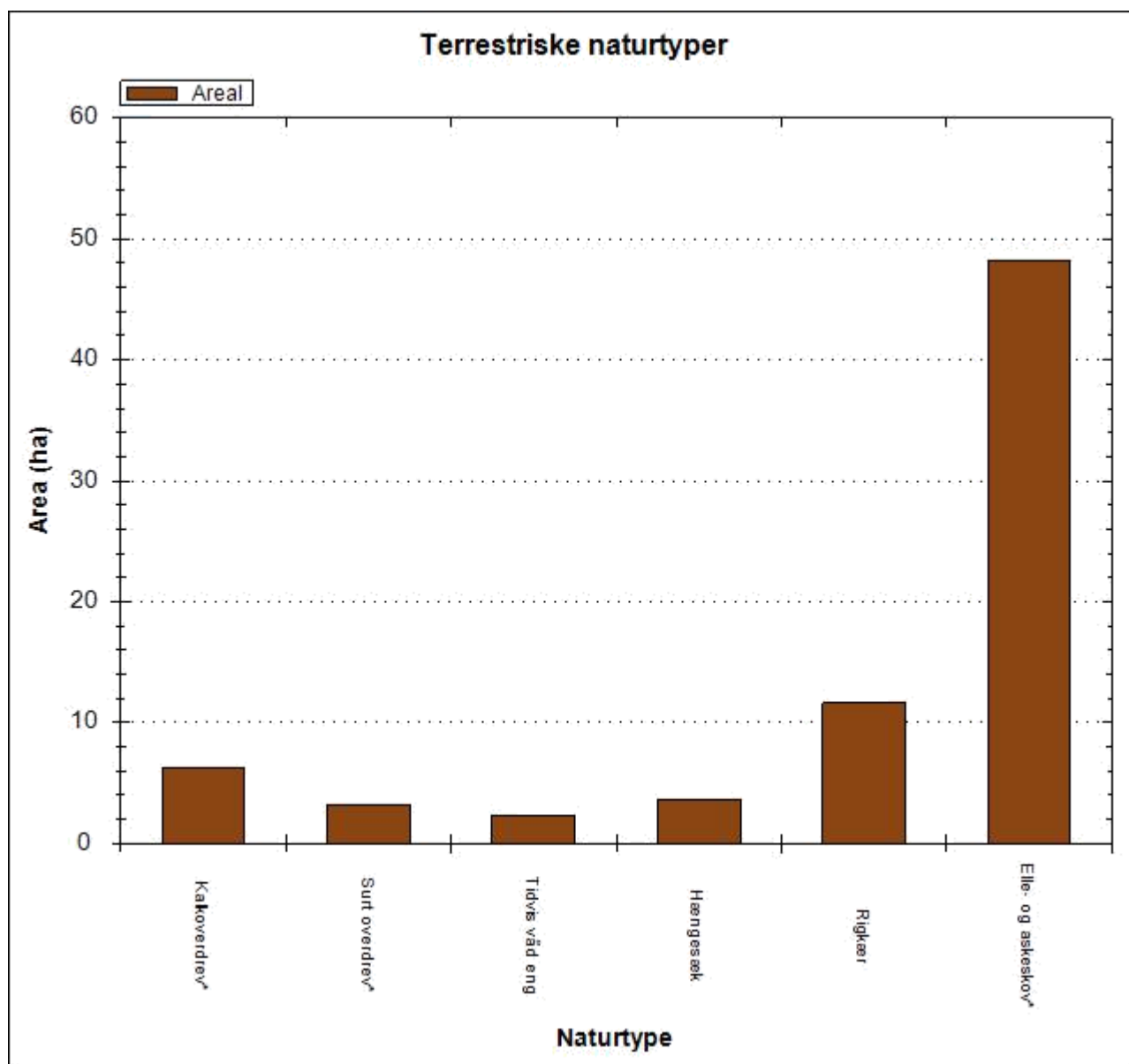
Areaifordelingen af områdets kortlagte naturtyper.
